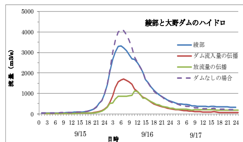
図 5 大野ダムの調節効果
